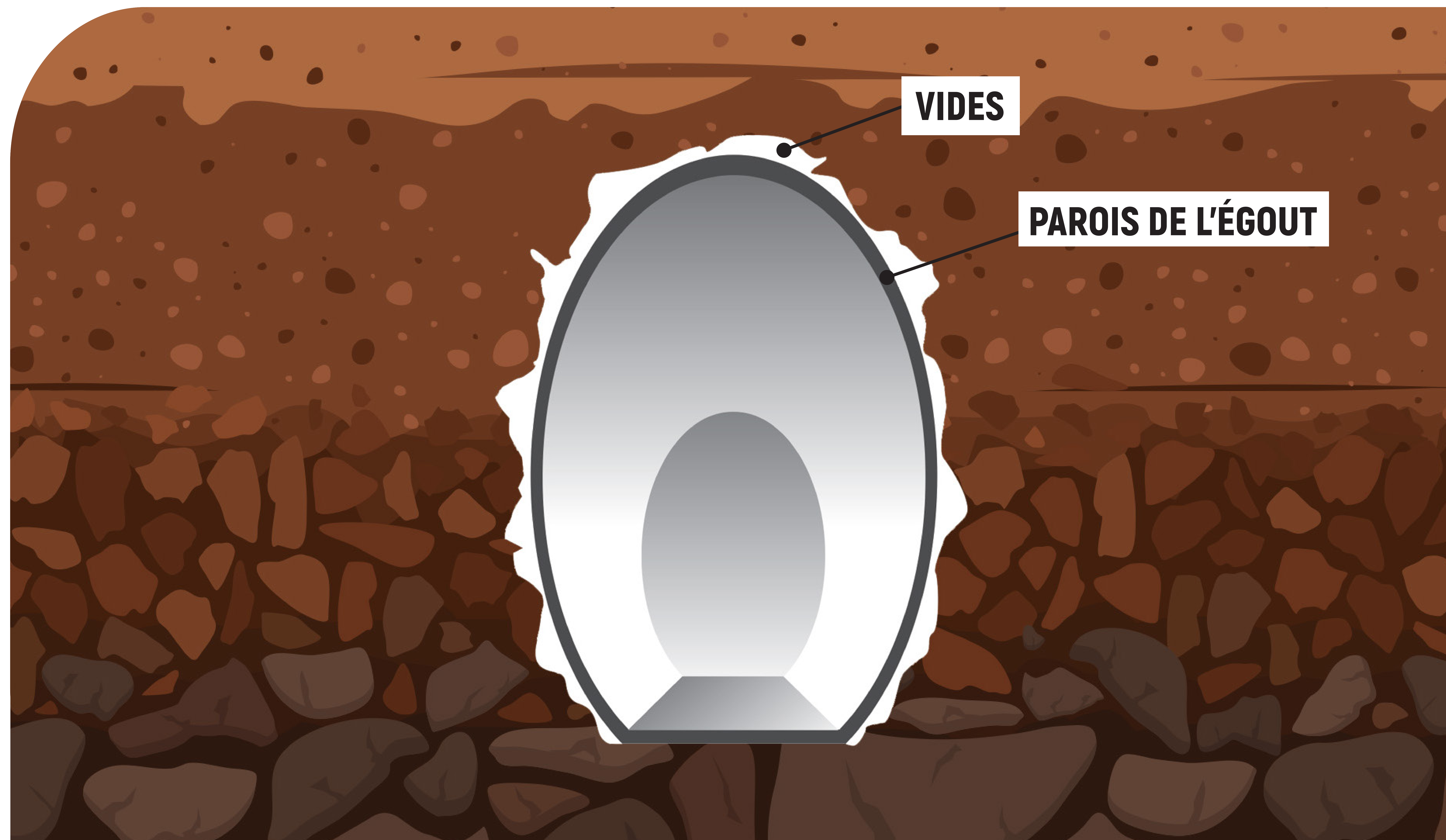
Schéma de coupe d'un égout avant réhabilitation
